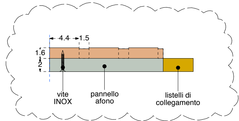
DETTAGLIO
